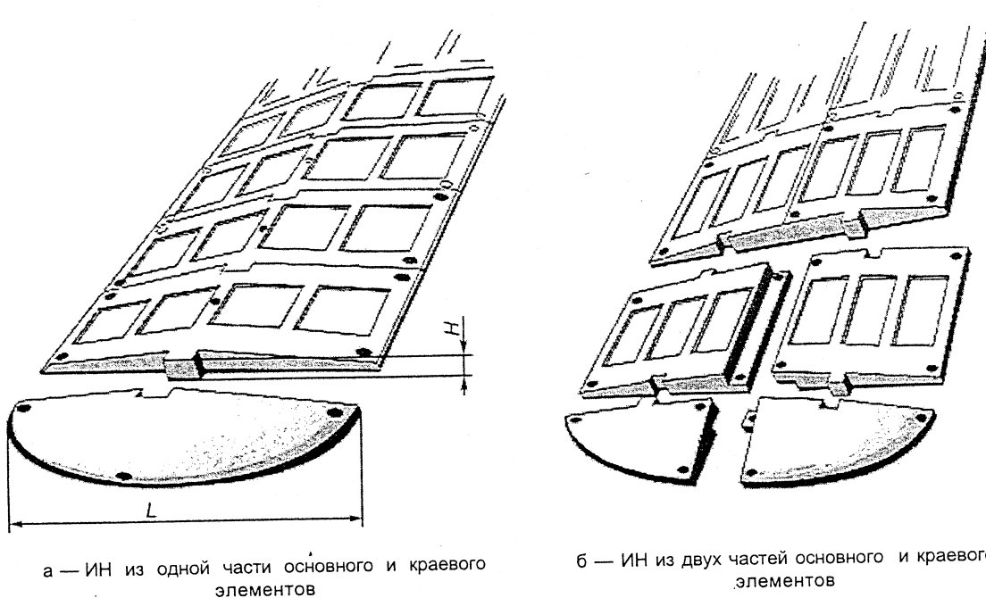
Рисунок 3 — Конструкция сборно-разборной ИН
